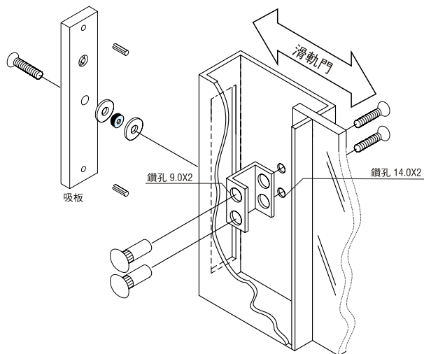
固定螺絲
