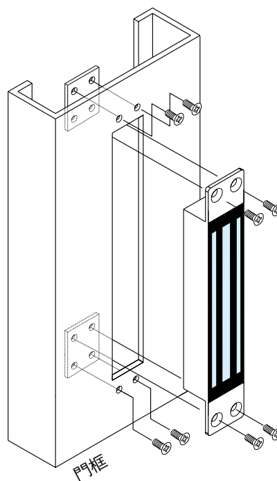
固定螺絲
